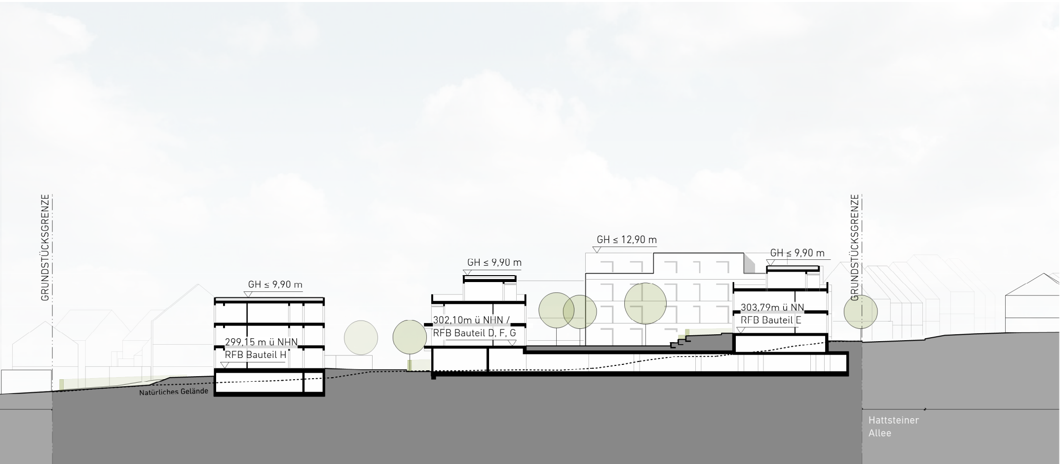
Schnitt A-A
