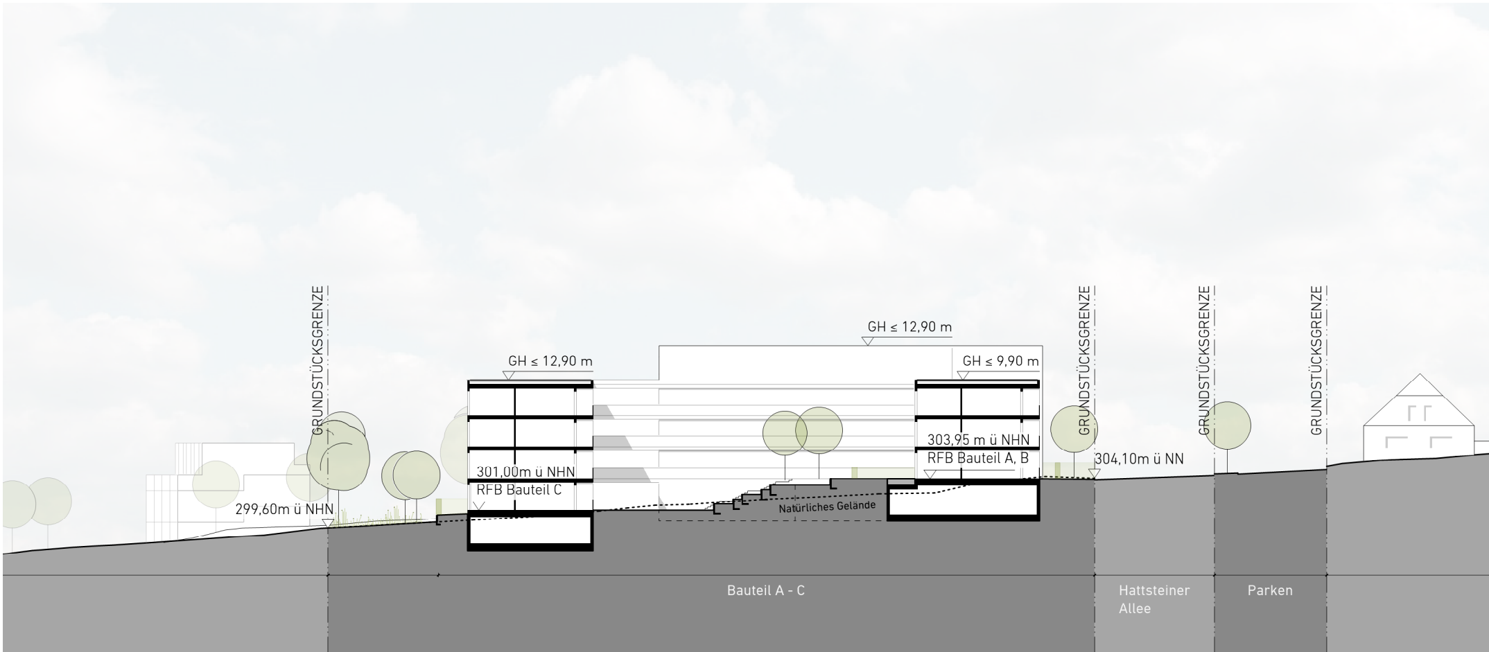
Schnitt B-B
