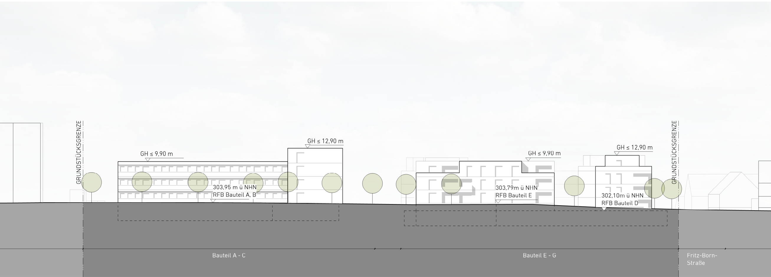
Ansicht Hattsteiner Allee
